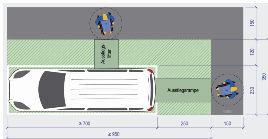
Bild 1 — Haltefläche (Maße in cm)
