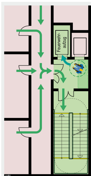
Bild A.1a — Sicherer Verweilbereich zwischen Feuerwehraufzug und Fluchttreppenhaus
