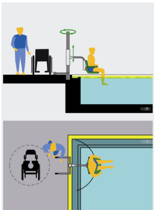
Bild 5a — Schwimmbadhebelift
