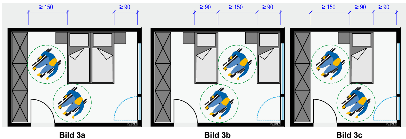
Bild 3 — Schlafräume (Maße in cm)
