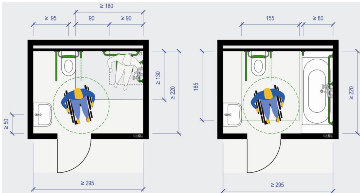
Bild 2 — Beispiel für Sanitärräume (Maße in cm)
