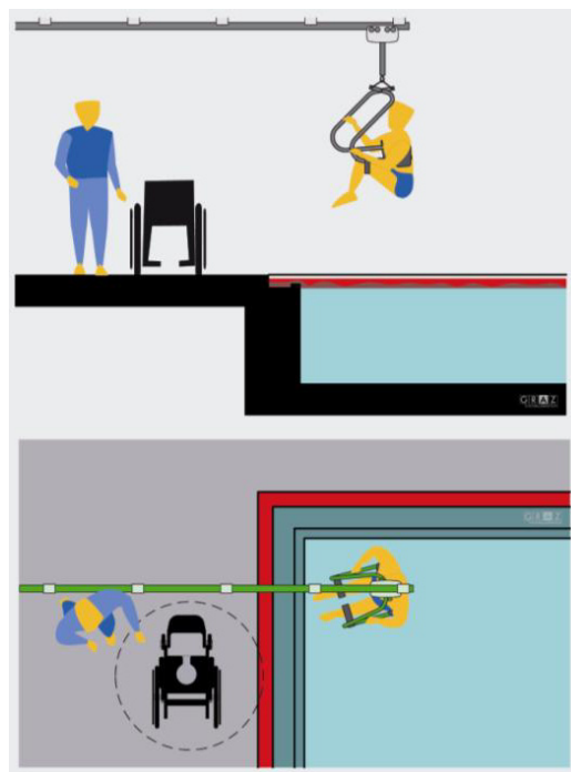
Bild 5b — Deckenschienenlifter
