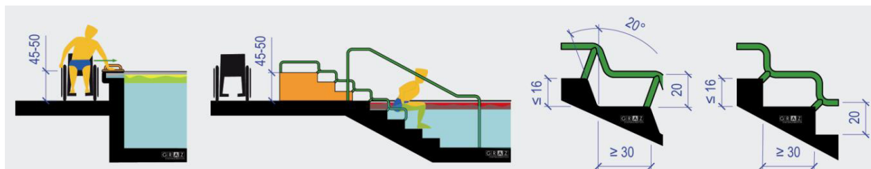
Bild 4a — Erhöhter Beckenrand
