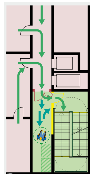
Bild A.1c — Erweiterung des Fluchttreppen- hauses mit einem sicheren Verweilbereich
